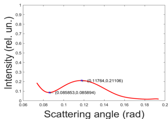
Угловое распределение интенсивности света в дифракционной картине
