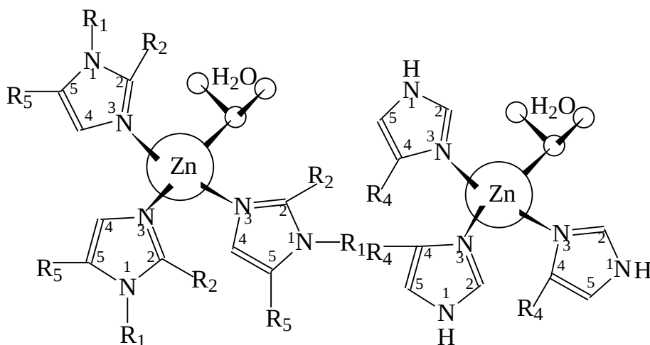
Рис1. Структура синтезированного комплекса метронидазола(а); Структура карбоангидразы С.
